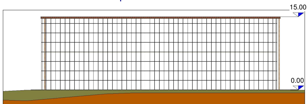
Coupe A - A : 1 : 500
